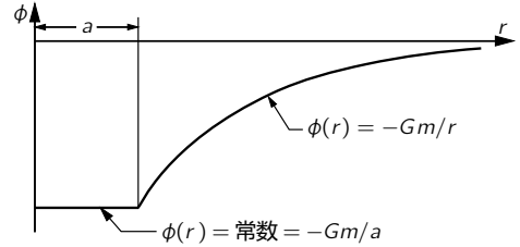
图 14.4: 由半径为 a 的球壳所引起的势能
